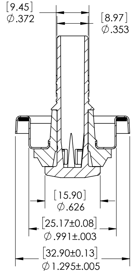
SECTION A-A
