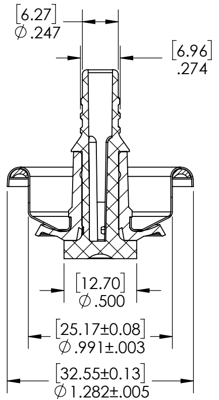
SECTION A-A
