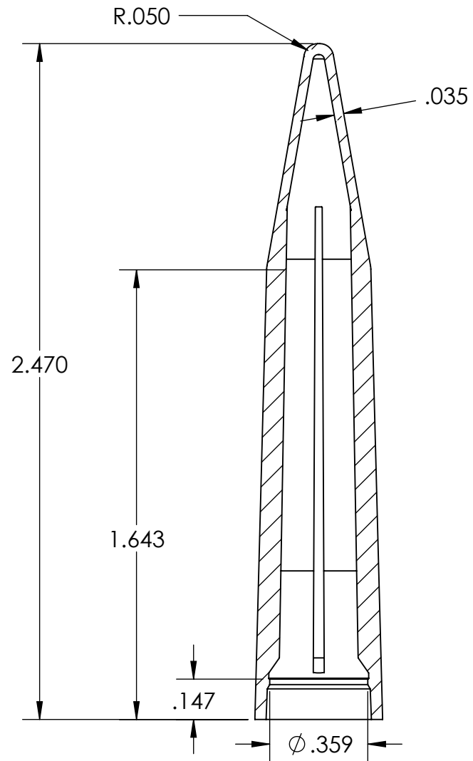
SECTION D-D
